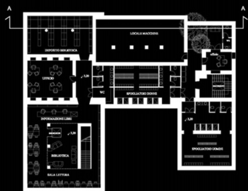
PLANIMETRIA QUOTA - 2.00 M
