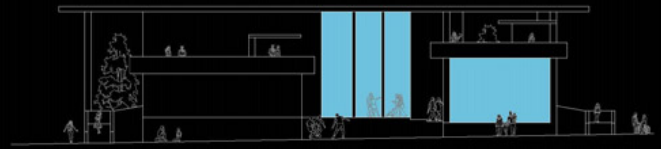
PROSPETTO NORD SCALA 1:200
